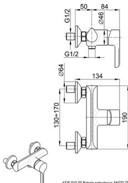
4726-010-00 Bateria natryskowa-ANGELIT
